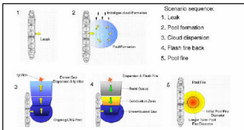
Figura 5 (tratta da [1]) – Scenari incidentali conseguenti a rilascio da nave
